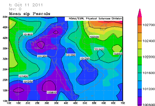
الگوی فشاری سطح زمین
